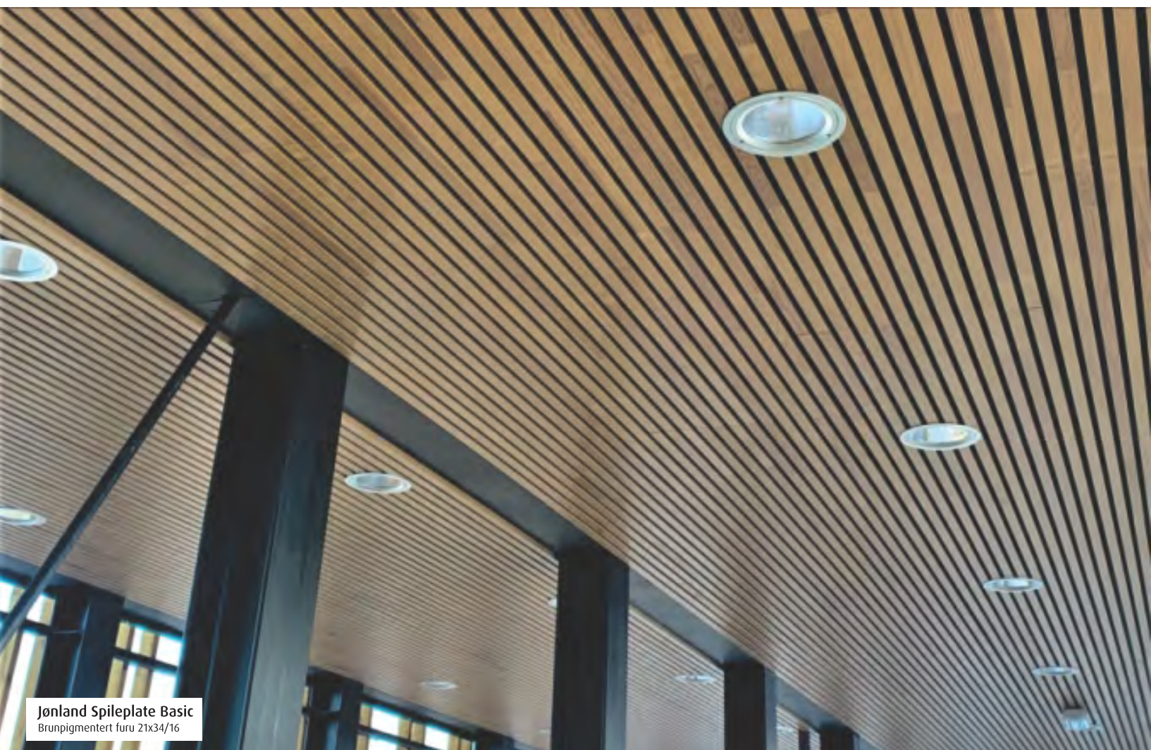
Jønland Spileplate Basic Hvitpigmentert furu 21x34/16
